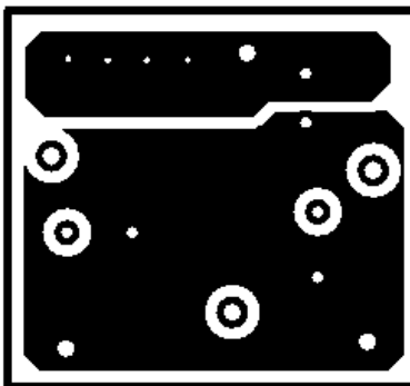
Fig. 10 Bottom layer of SO-8
