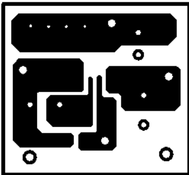
Fig. 9 Top layer of SO-8
