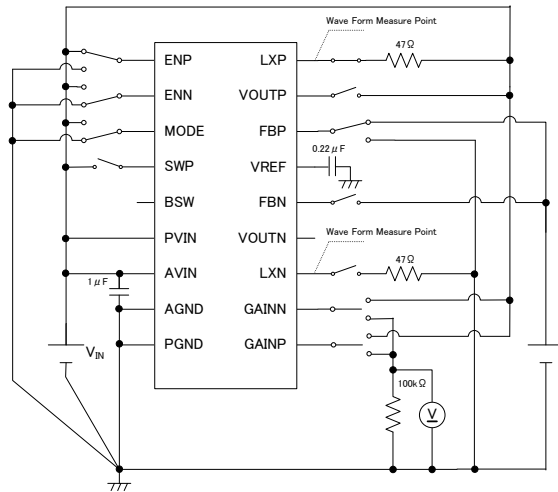
4) Circuit
