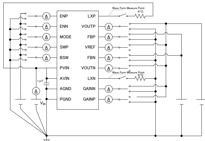
7) Circuit ⑦
