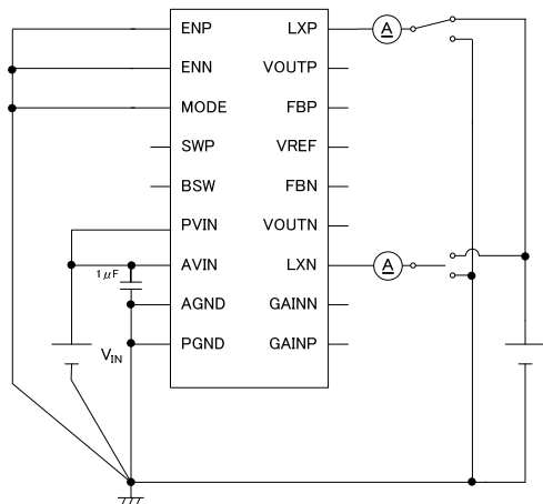
7) Circuit ⑦
