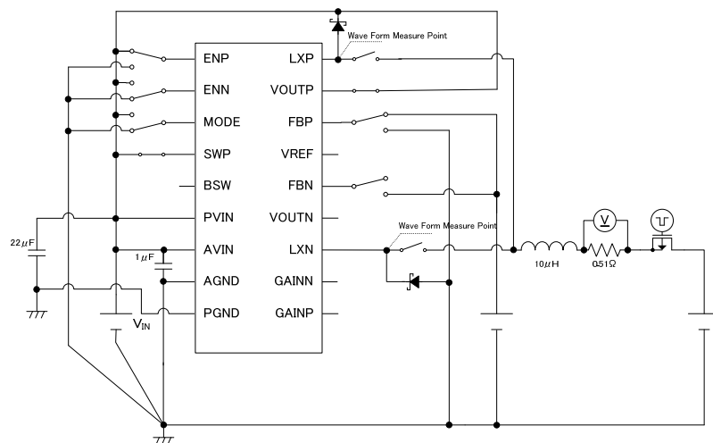
6) Circuit
