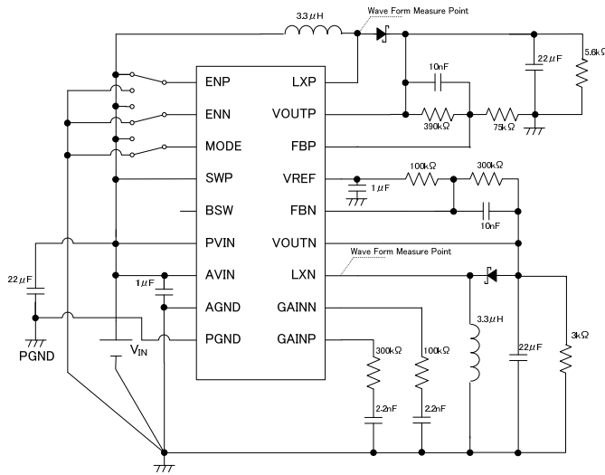
9) Circuit ⑨
