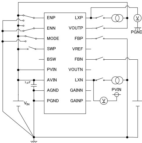
4) Circuit
