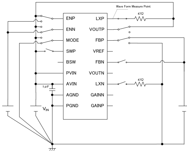
9) Circuit ⑨
