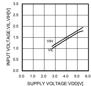
Fig.17 Input voltage
