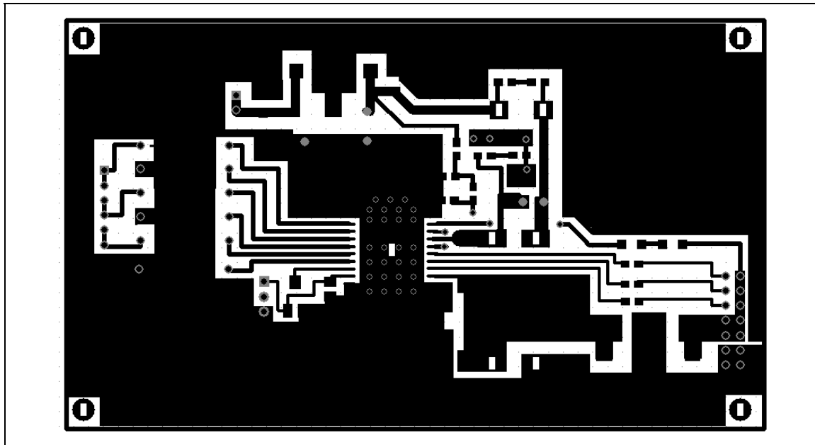
Figure 18 : PBC Bottom Layer
