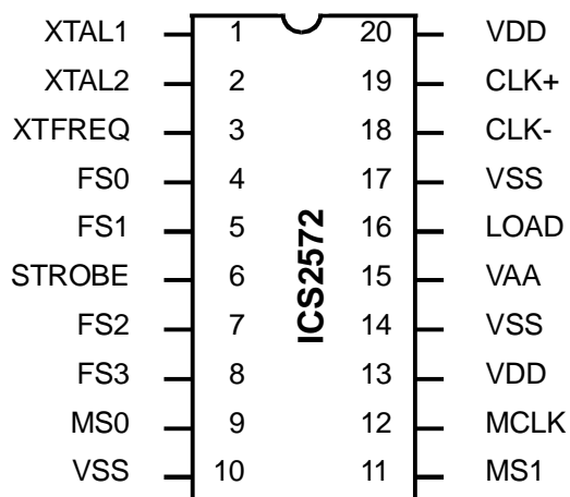
20-Pin DIP or SOIC J-4, J-7
