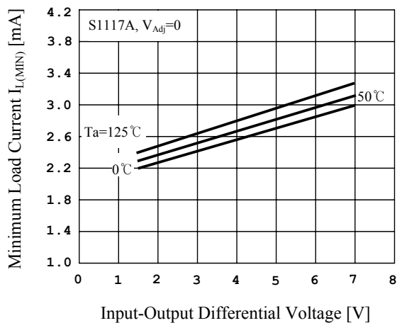
Fig.5 I_{L(MIN)} vs V_I - V_O
