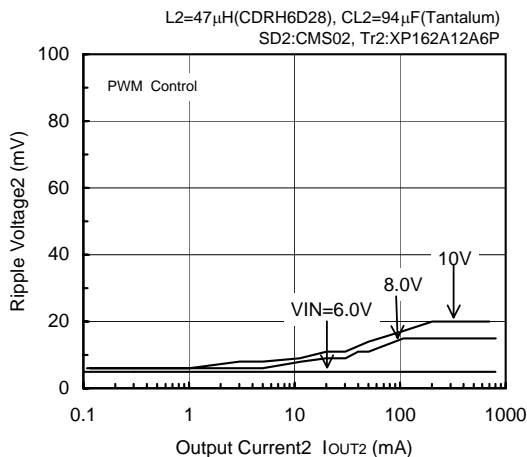
FOSC=180kHz, VOUT2=5.0V
