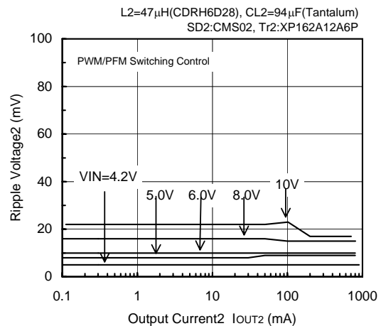
FOSC=180kHz, VOUT2=5.0V
