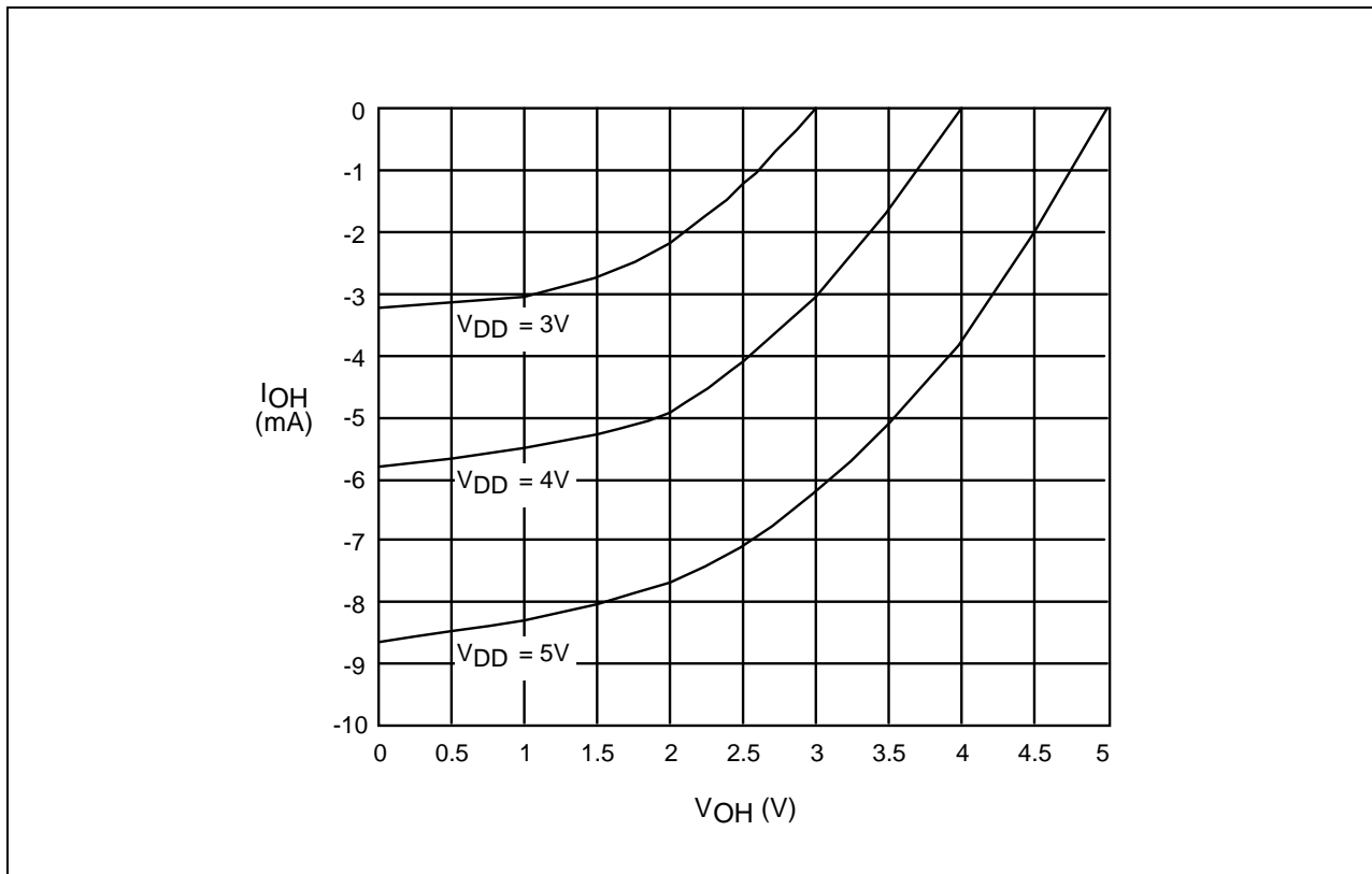
Figure 14-6. I_{OH} vs. V_{OH} (Port 0)
