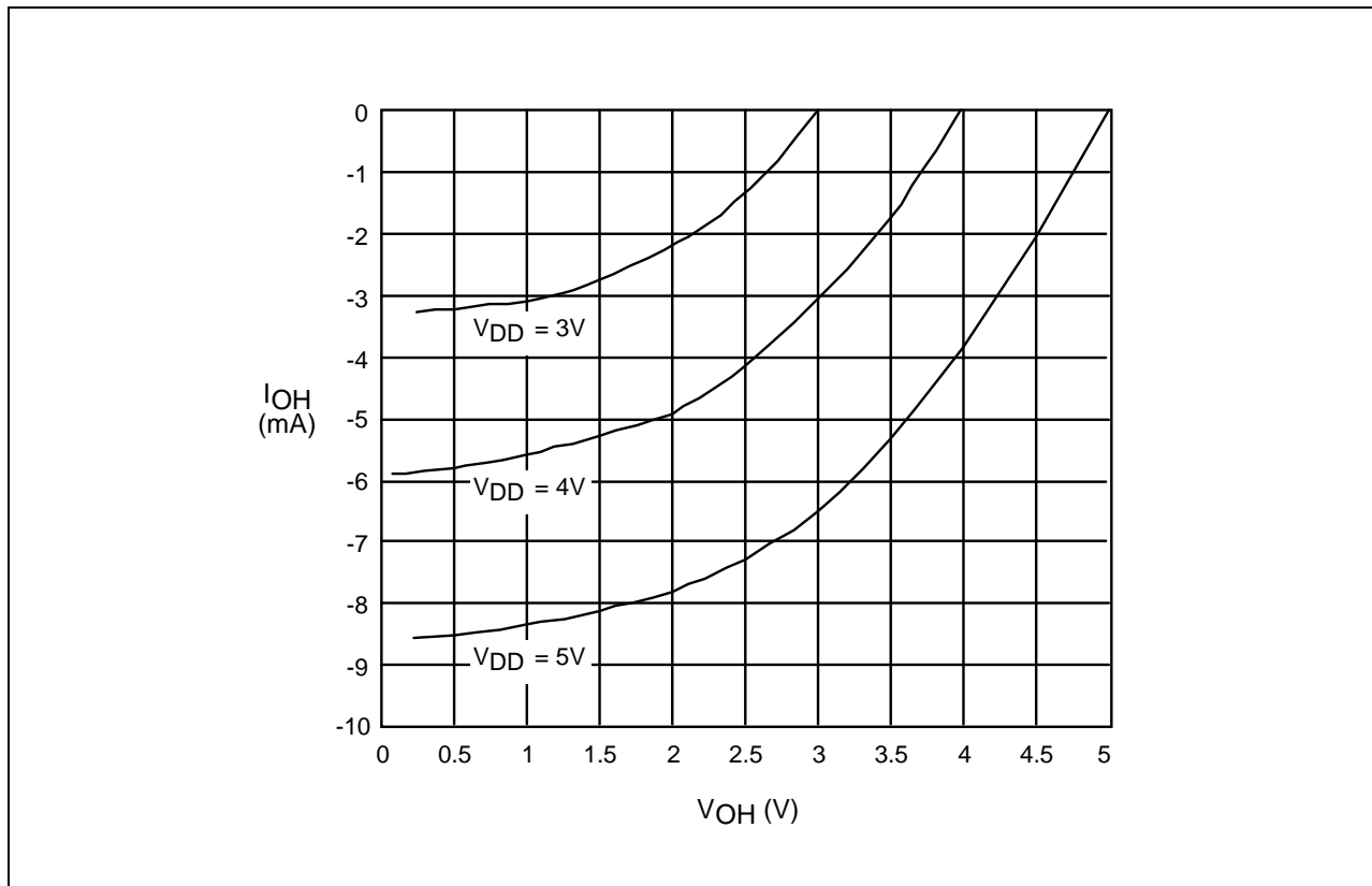
Figure 14-7. I_{OH} vs. V_{OH} (Port 2)
