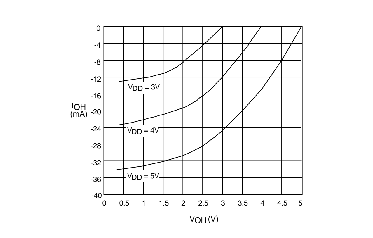
Figure 14-8. I_{OH} vs. V_{OH} (Port 3)
