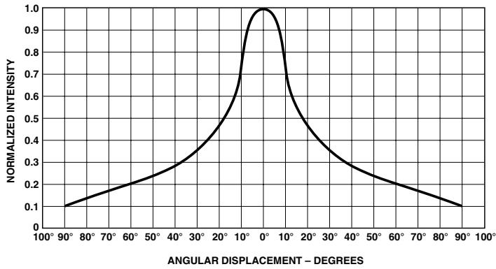
Figure 9. HLMP-Q102/-Q152
