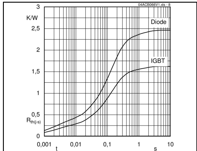
Fig. 8 Thermal impedance
