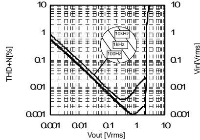
Fig.2 Thd vs Vo
