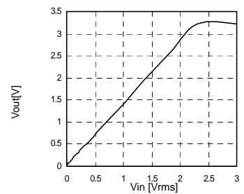
Fig.21 Level Meter Vin vs Vo
