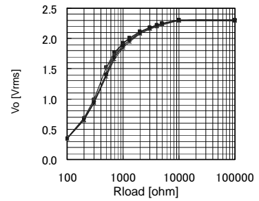
Fig.18 Rload vs Vo
