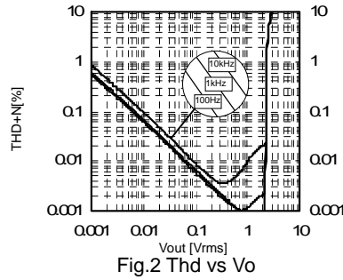
Fig.2 Thd vs Vo
