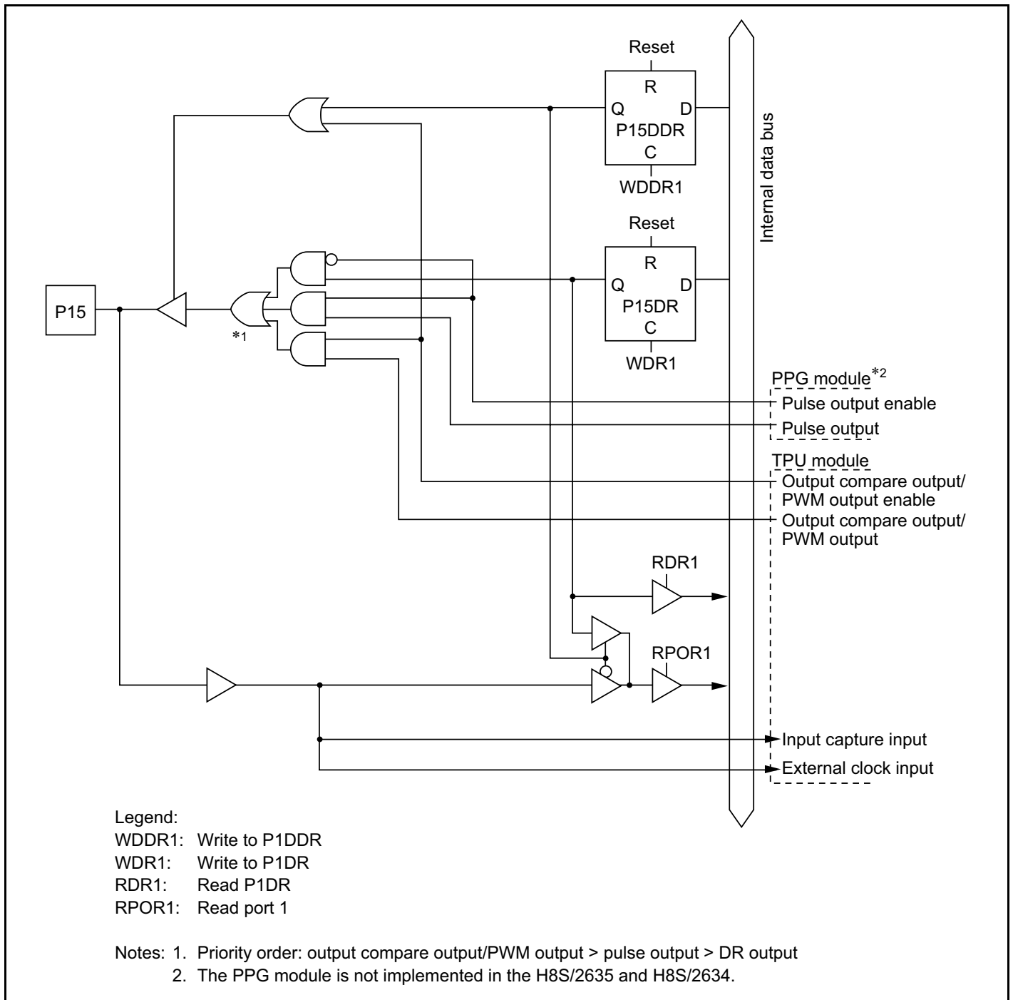
Figure C-1 (d) Port 1 Block Diagram (Pin P15)
