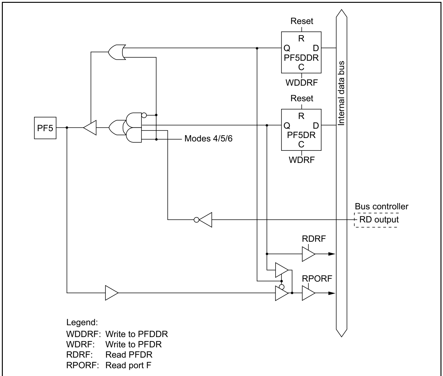
Figure C-10 (d) Port F Block Diagram (Pin PF5)
