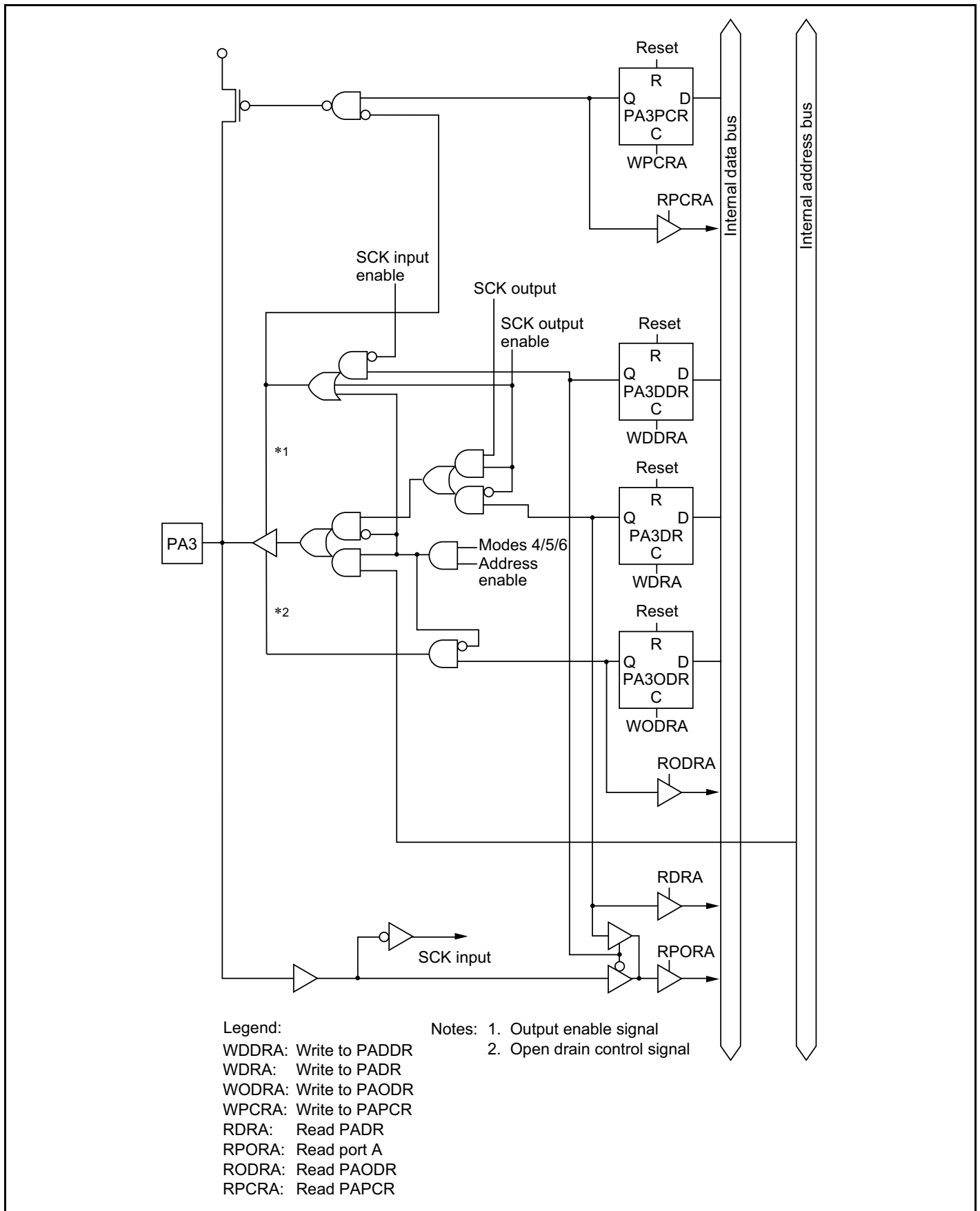
Figure C-5 (d) Port A Block Diagram (Pin PA3)
