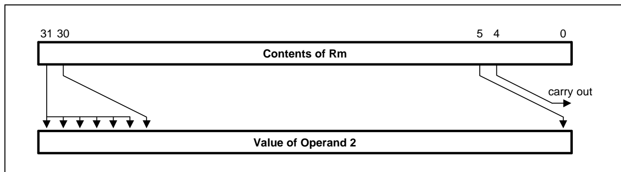
Figure 3-8. Arithmetic Shift Right
