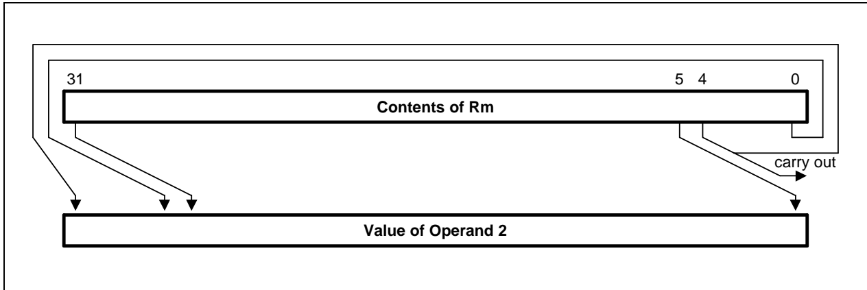
Figure 3-9. Rotate Right
