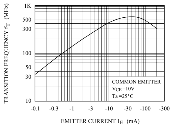
f_T - I_E
