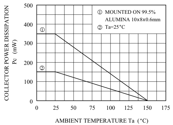
P_c - T_a
