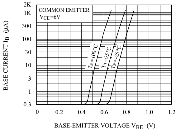
I_B - V_{BE}
