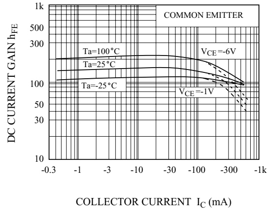
h_{FE} - I_C
