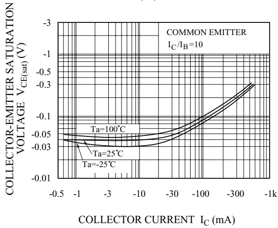
V_{CE(sat)} - I_C
