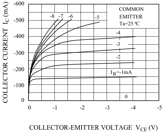
I_C - V_{CE}
