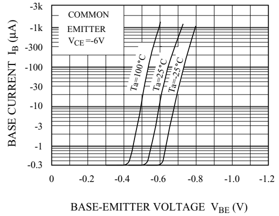
I_B - V_{BE}
