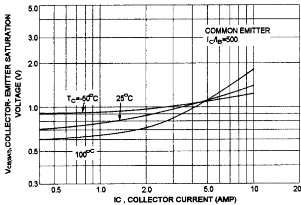
V_{CE(sat)} - I_C
