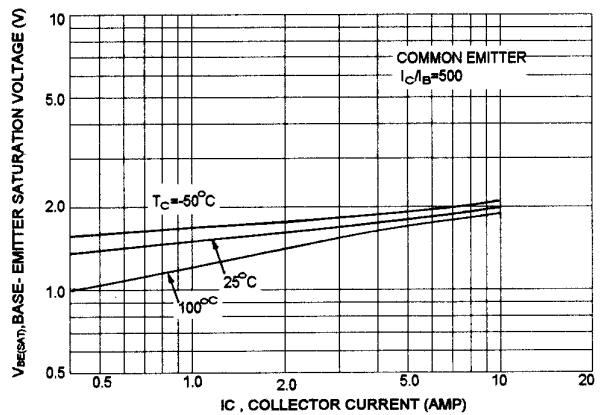
V_{BE(sat)} - I_C
