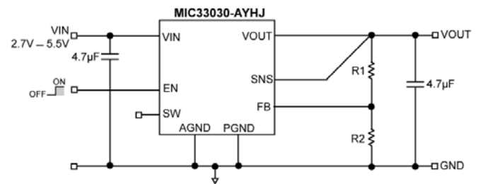
Figure 1. MIC33030-AYHJ Schematic
