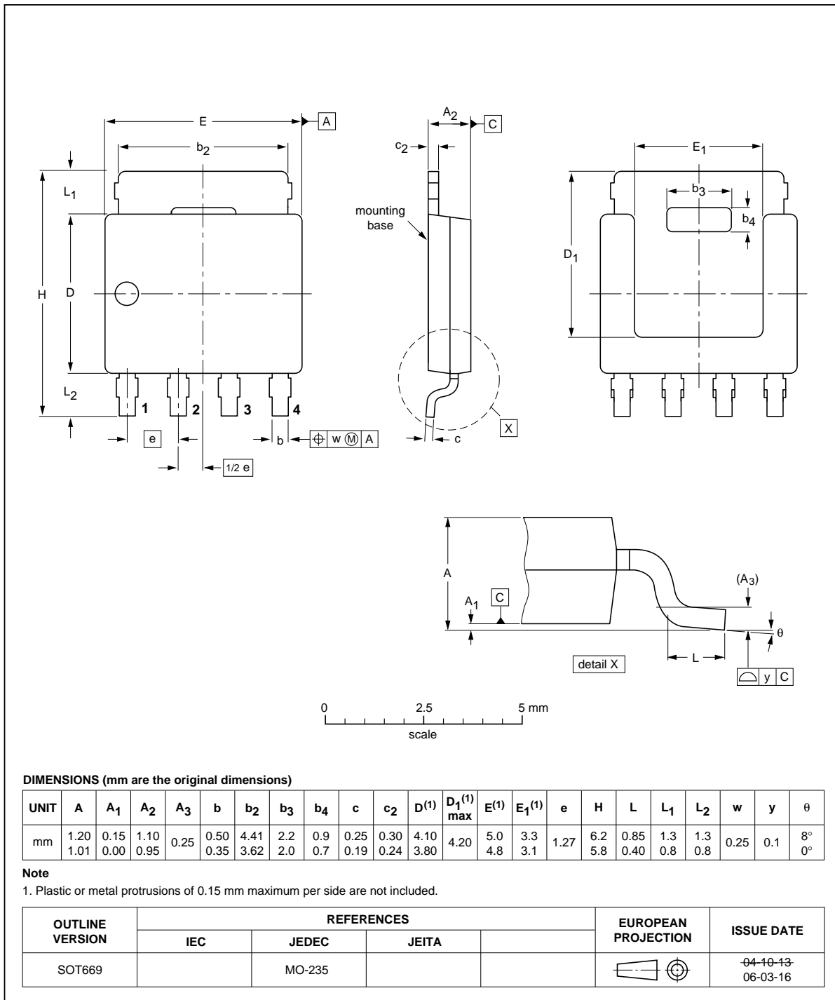
Fig 21. Package outline SOT669 (LFPAK)
