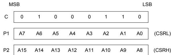
Figure 6-22: CSRW Parameters
