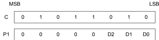
Figure 6-20: HDOT SCR Parameters
