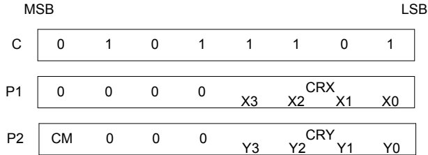
Figure 6-13: CSRFORM Parameter Bytes
