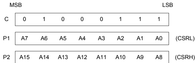
Figure 6-23: CSRR Parameters
