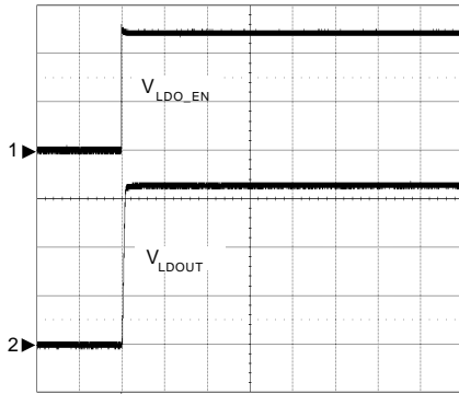
LDO Enable
