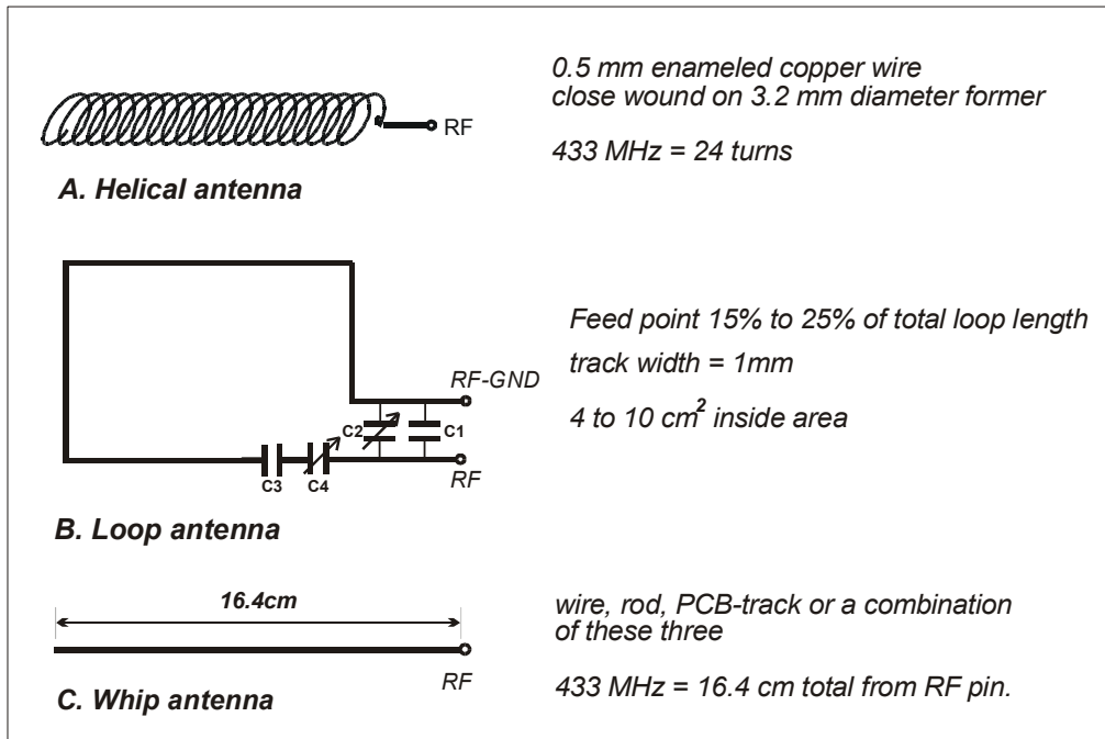
Fig. 7: Antenna
