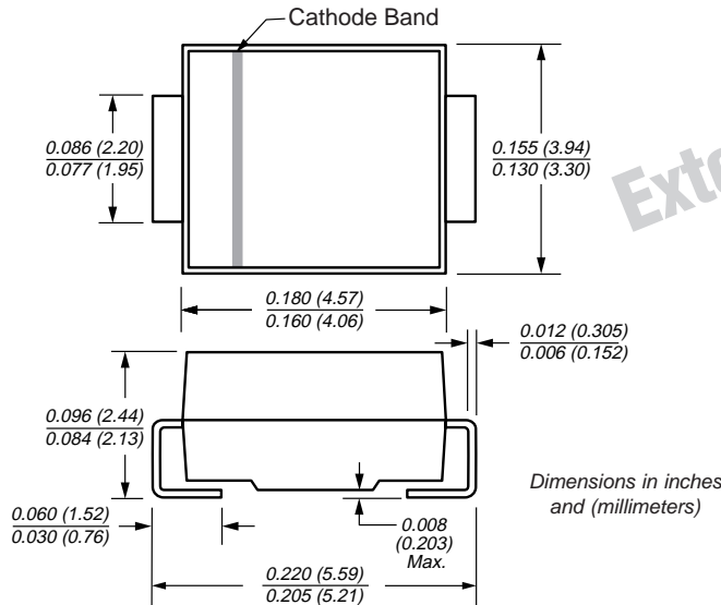
DO-214AA (SMBJ-Bend)
