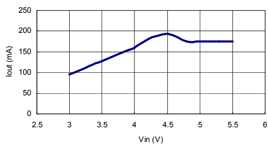
Vin & Iout
