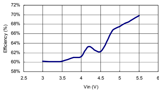
Vin & Efficiency
