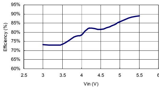
Vin & Efficiency
