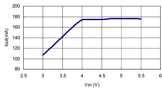
Vin & Iout
