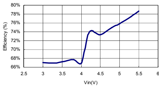
Vin & Efficiency
