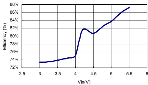
Vin & Efficiency
