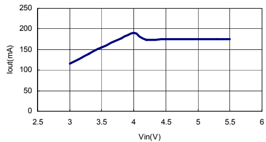
Vin & Iout
