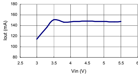
Vin & Iout
