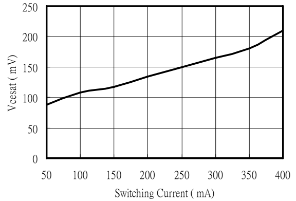
Vcesat
