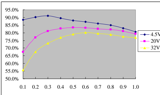
Vo = 1.8V
