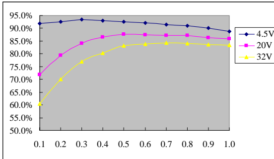
Vo = 3.3V
