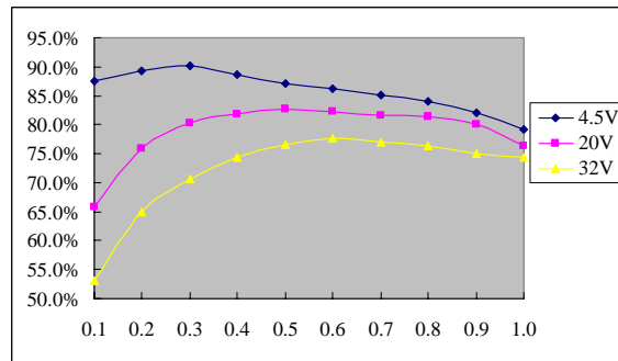
Vo = 1.5V
