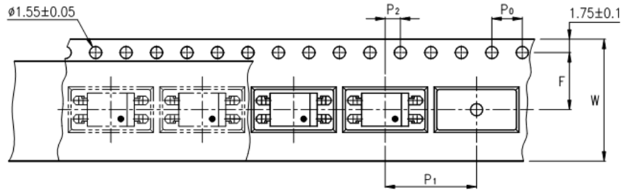
LTV-817S-TA :
