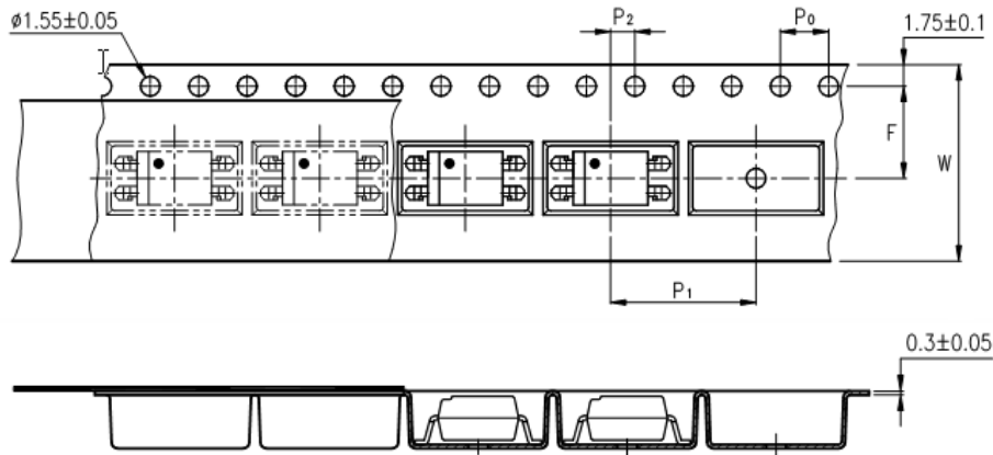
LTV-817S-TA1 :
