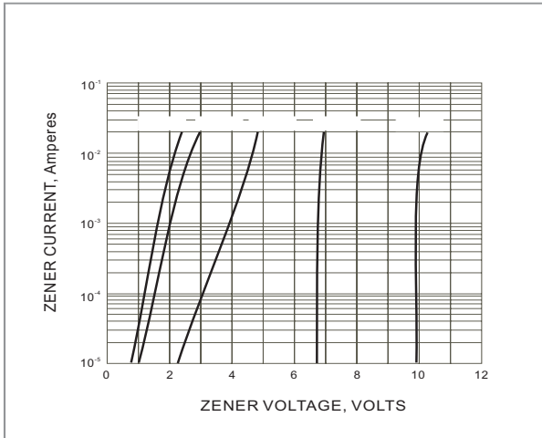
Fig.7 ZENER VOLTAGE VERSUS ZENER CURRENT
