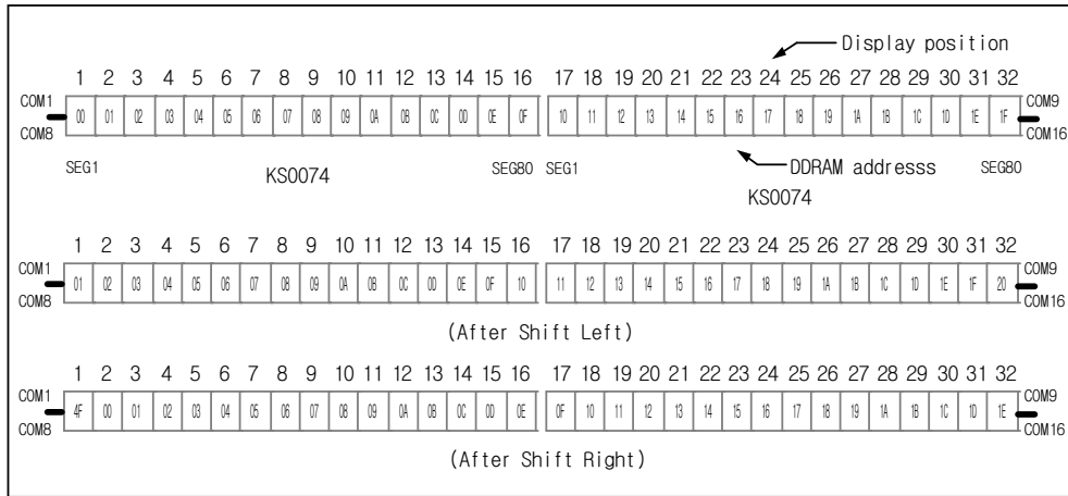
Fig-2. 1-line X 32ch. display
