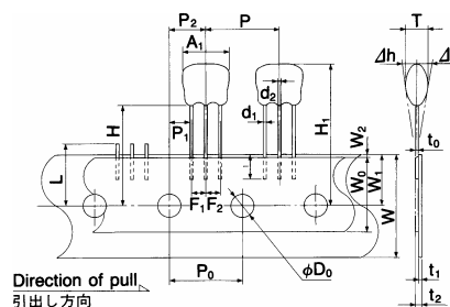
CFSKP/CFSCP Dimensions
