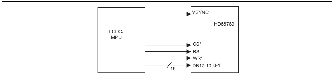
VYSNC interface
