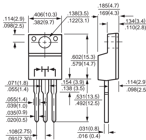
ITO-220
