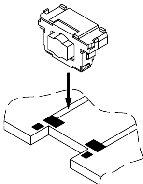
Fig.1 Edge Mounting
