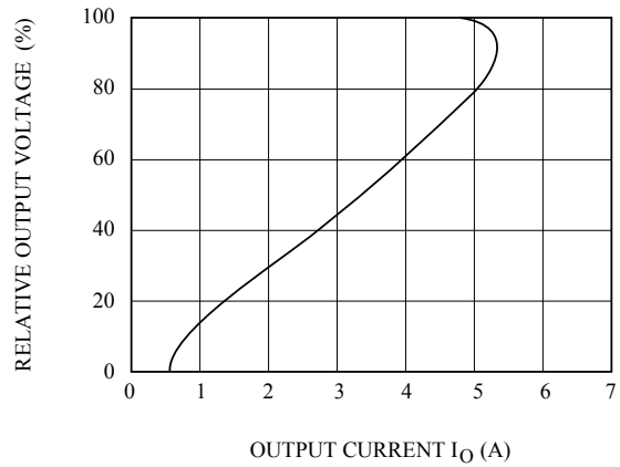
Fig.4 I_O - V_O
