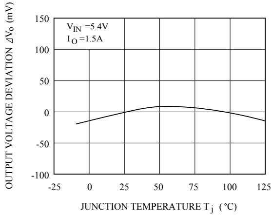
Fig.5-1 T_j - \Delta V_o (KIA378R37)
