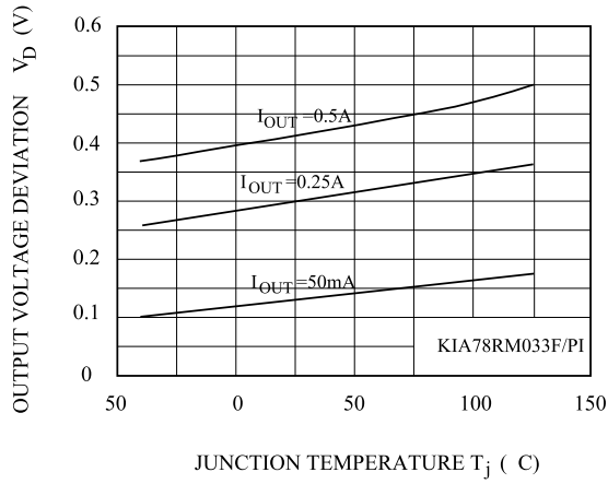
Fig.12 V_D - T_j
