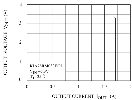
Fig. 11 V_{OUT} - I_{OUT}
