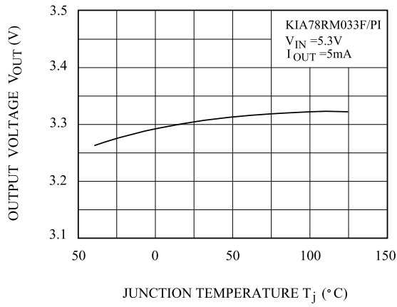
Fig. 6 V_{OUT} - T_j
