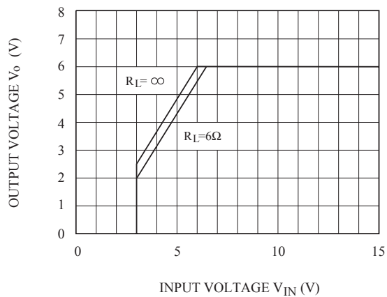
Fig.6-2 V_{IN} - V_o (KIA78R06)
