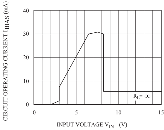
Fig.7-3 V_{IN} - I_{BIAS} (KIA78R08)
