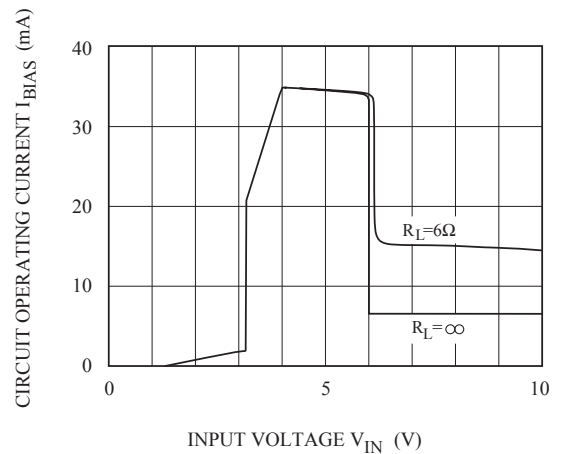
Fig.7-2 V_{IN} - I_{BIAS} (KIA78R06)
