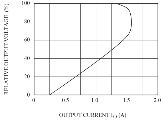
Fig.4 I_O - V_O
