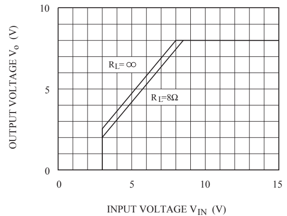
Fig.6-3 V_{IN} - V_o (KIA78R08)
