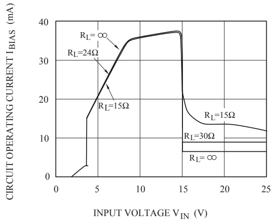
Fig.7-7 V_{IN} - I_{BIAS} (KIA78R15)
