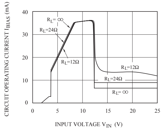
Fig.7-6 V_{IN} - I_{BIAS} (KIA78R12)
