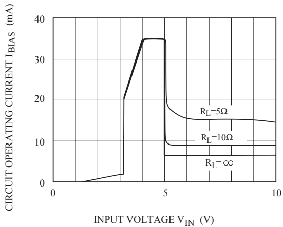
Fig.7-1 V_{IN} - I_{BIAS} (KIA78R05)
