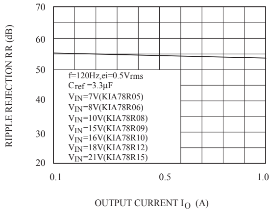
Fig.10-2 I_O - RR
