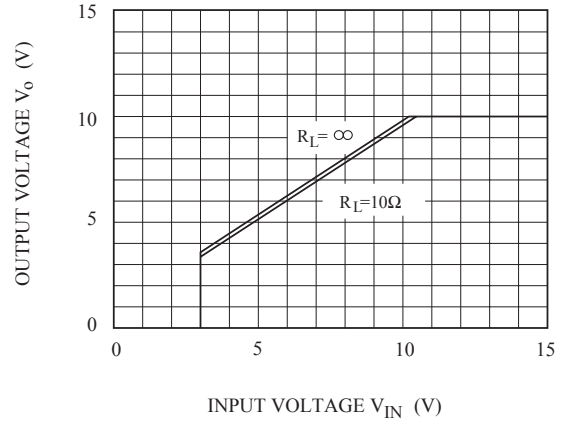
Fig.6-5 V_{IN} - V_o (KIA78R10)
