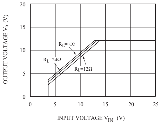
Fig.6-6 V_{IN} - V_o (KIA78R12)
