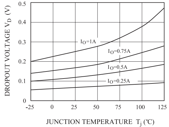
Fig. 7 V_D - T_j
