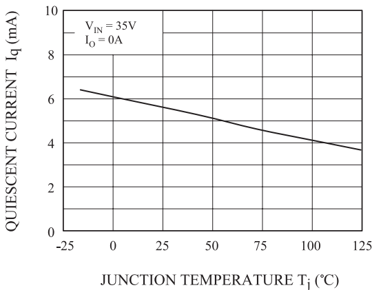
Fig. 8 I_q - T_j
