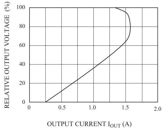
Fig. 5 V_{OUT} - I_{OUT}
