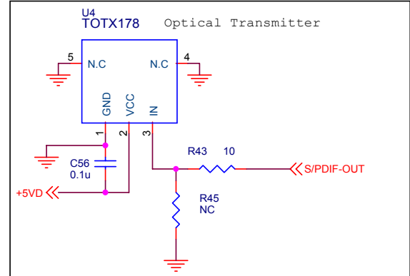
Figure 21. Optional SPDIF Output
