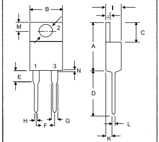
TO-220A
