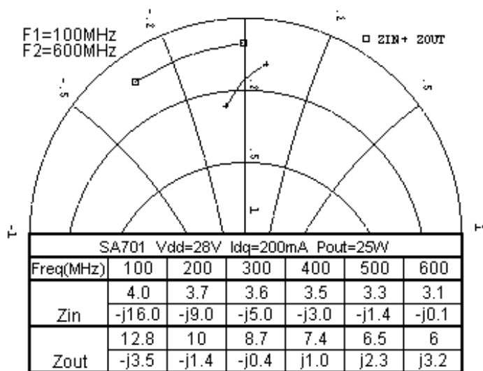
Zin Zout
