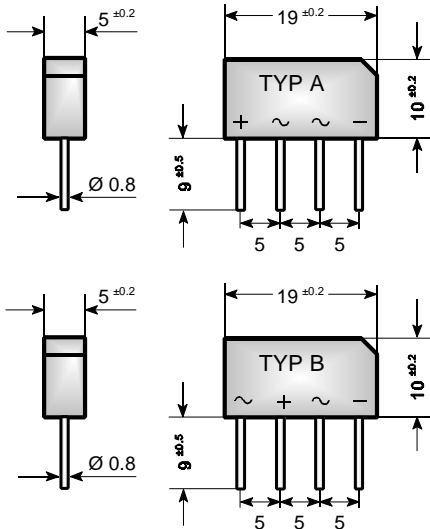
Dimensions / Maße in mm
