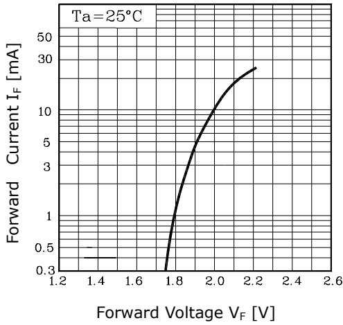
Fig. 1 I_F - V_F
