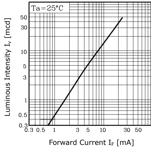
Fig. 2 I_V - I_F
