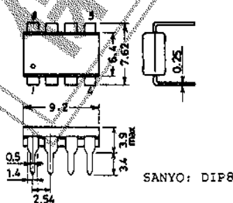
LA5521D 外形図 3001A-D8IC (unit: mm)
