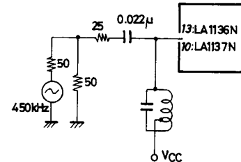
Detector input
