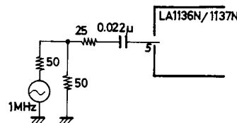
Mixer input
