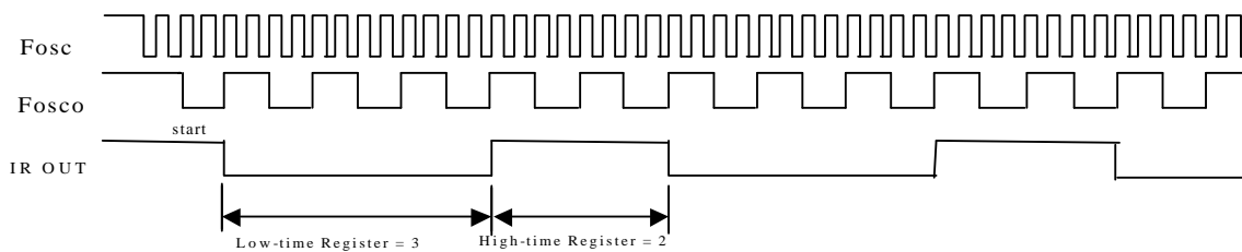
Fig. 30 Continuous pulse train (DP=00;MF=10;HF=0;LGP=0;PWM==1).
