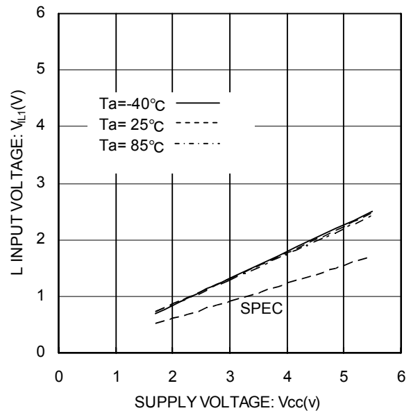
Fig.5 'L' input voltage V_{IL1} (A0,A1,A2,SCL,SDA,WP)
