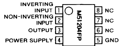
Outline 8P2S-A
