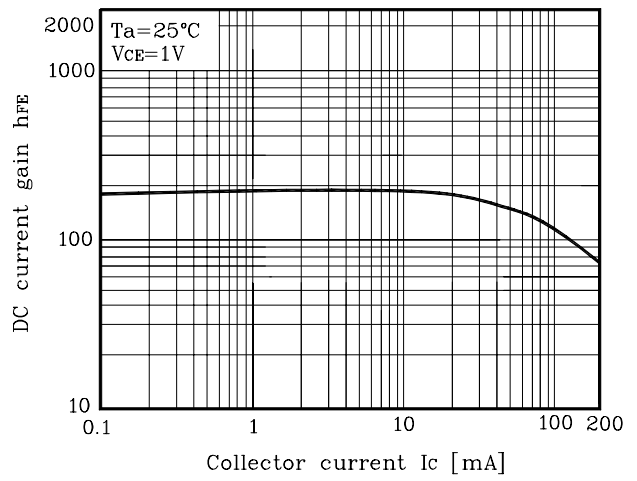
Fig. 2 h_{FE}-I_C
