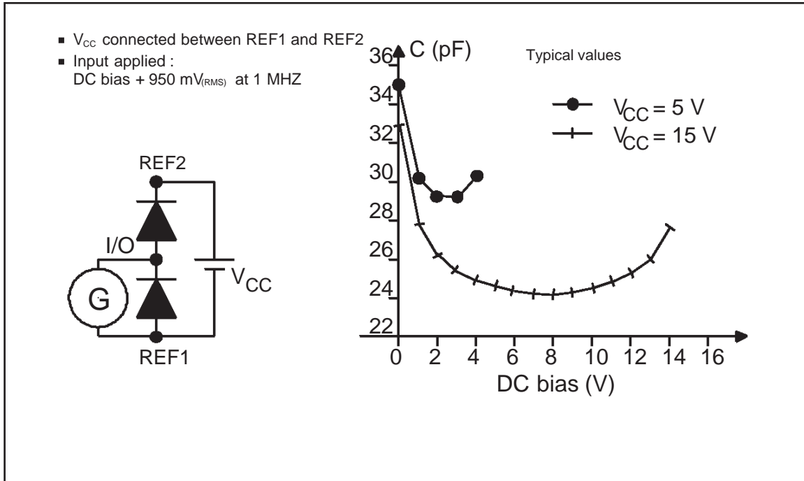
Fig.1 : Input capacitance
