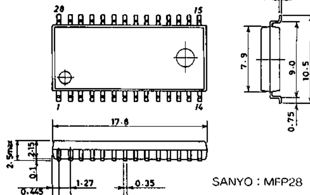
外形図 3091-M28IC [LC7883M]
