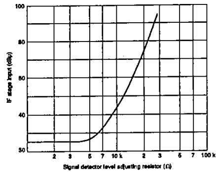
Figure 16. IF input vs. R_{SD \text{ de } j}
